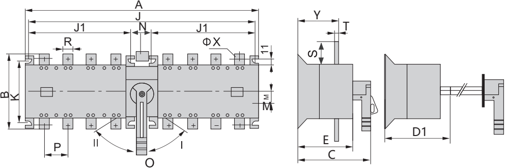
RDH5Z2-125A-630A柜内操作
