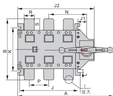
RDH5Z1-800A~1600A柜内操作
