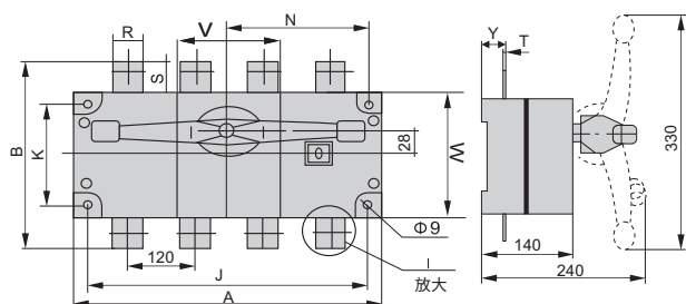
RDH5-800A-1600A系列隔离开关外形及安装尺寸
