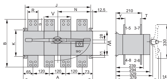
RDH5-2000A-3200A柜内操作
