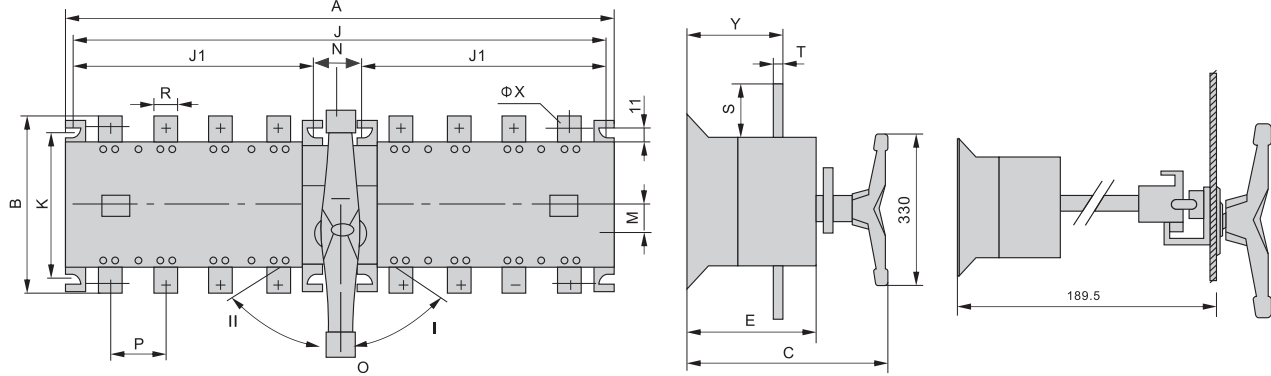
RDH5Z2-800A~1600A柜内操作
