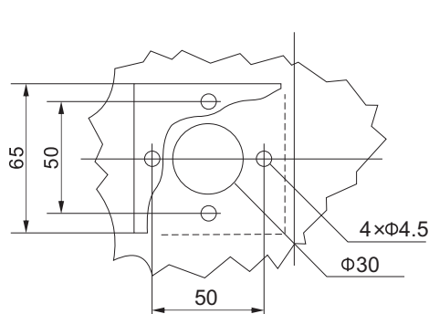
柜外手柄座安装尺寸
