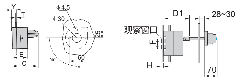
柜外手柄座安装尺寸
