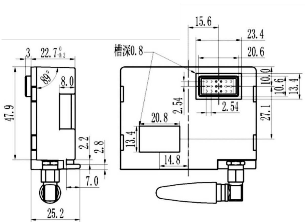
图A.5 集中器远程通信模块（无线）外形结构和尺寸示意图
