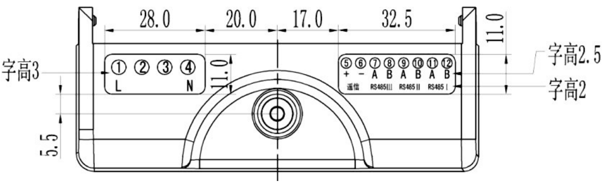
图 A. 4 集中器接线端子标识位置示意图
