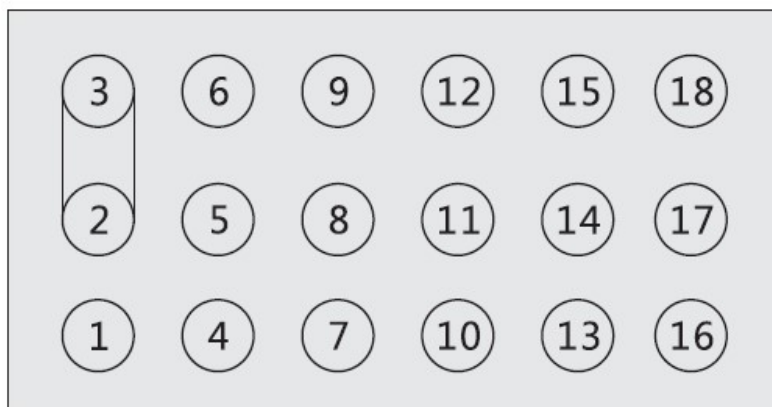
图1 集中器远程通信模块接口定义（俯视）
